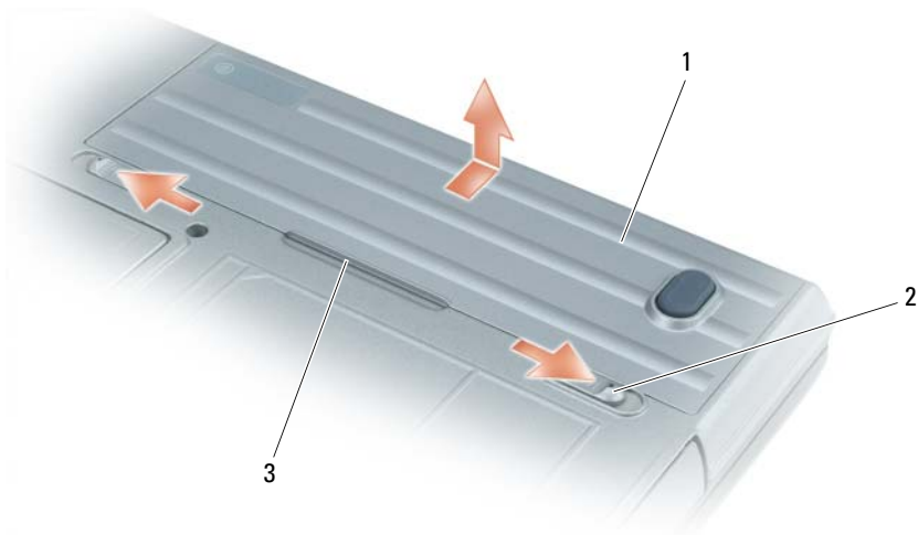
1 电池 2 电池槽释放闩锁（2个） 3 电池卡舌
